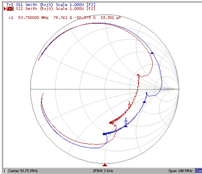
Диаграмма Смита
