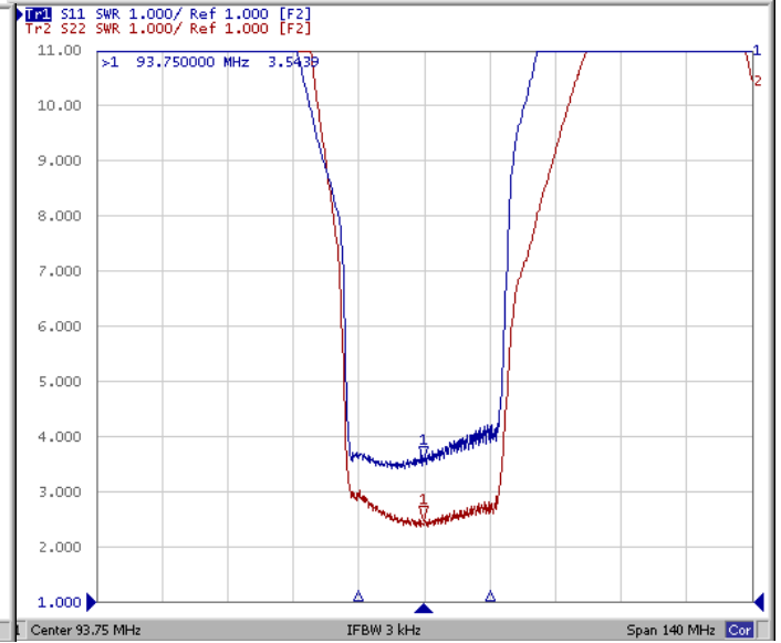
КСВ
