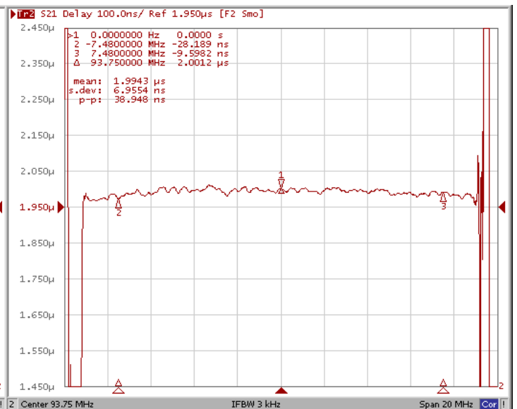
Неравномерность ГВЗ
