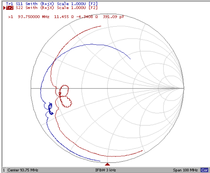
Диаграмма Смита
