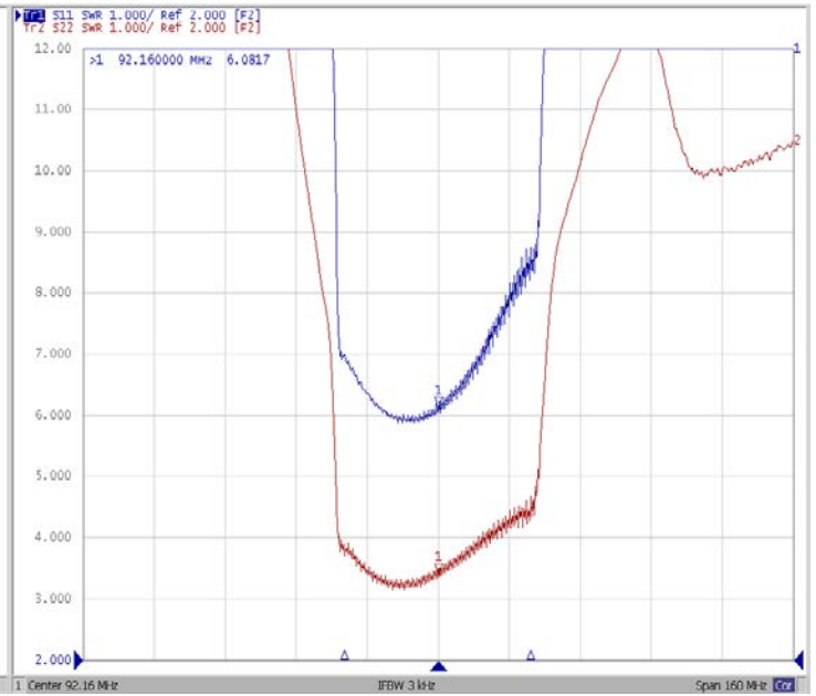
КСВ
