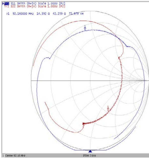
Диаграмма Смита
