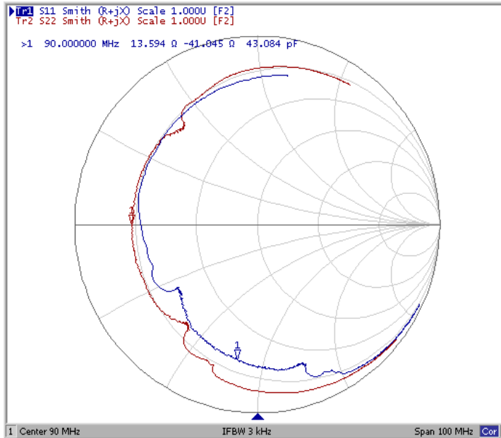
Диаграмма Смита
