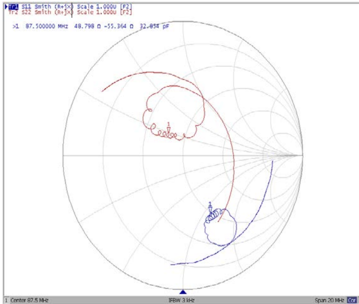
Диаграмма Смита
