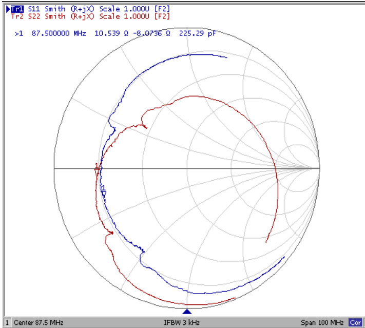
Диаграмма Смита
