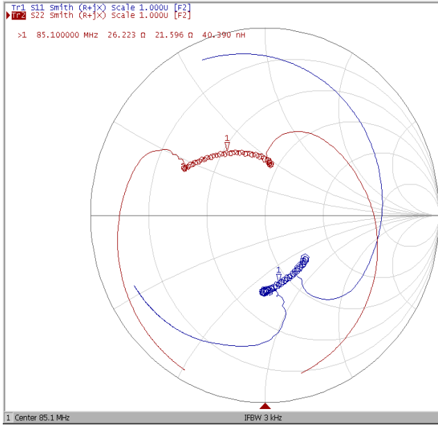
Диаграмма Смита
