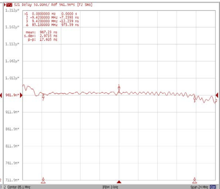
Неравномерность ГВЗ
