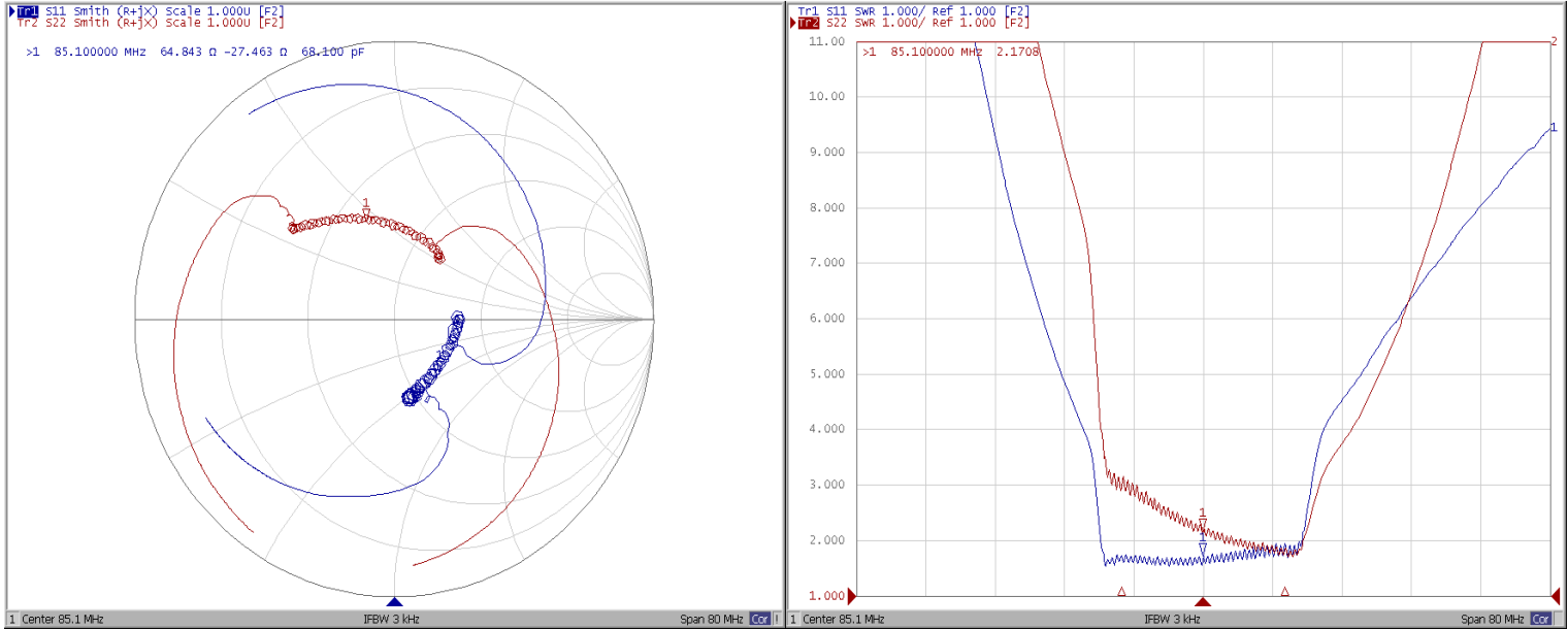
Диаграмма Смита
