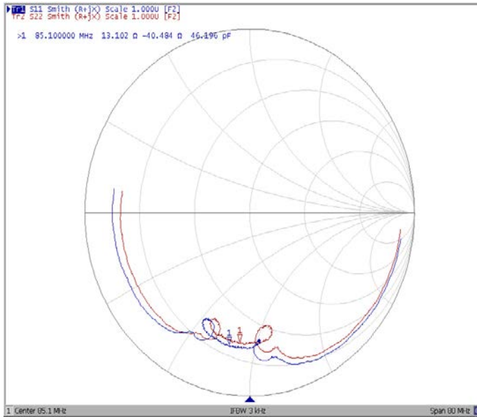
Диаграмма Смита
