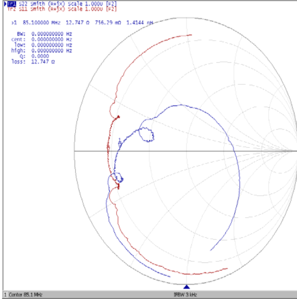
Диаграмма Смита
