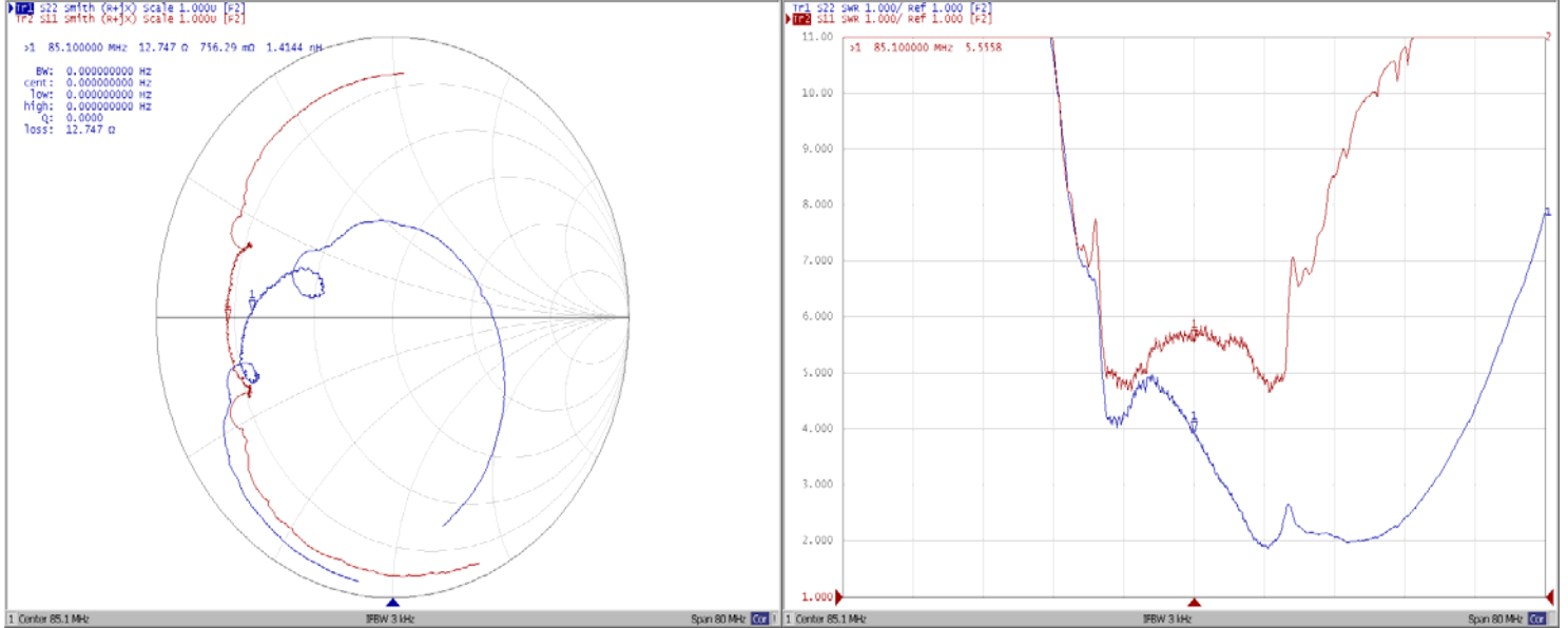
Диаграмма Смита
