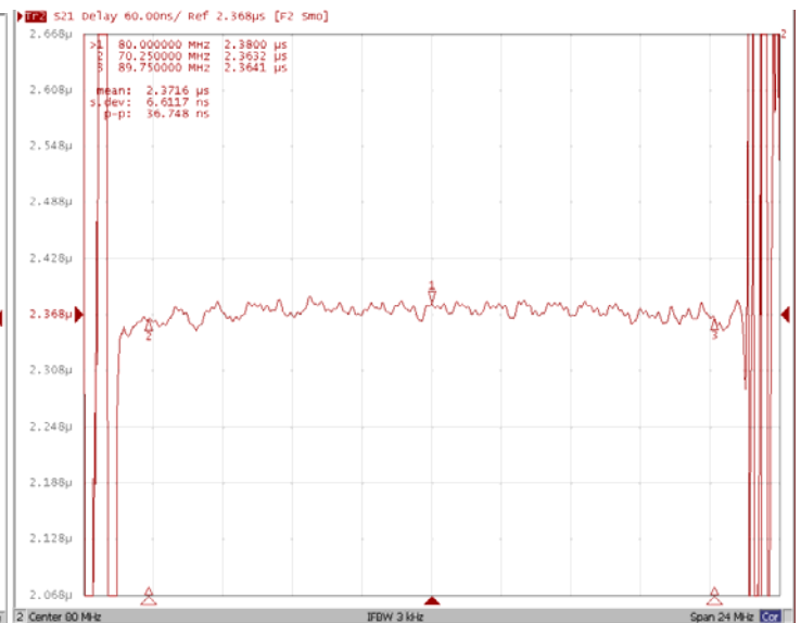
Неравномерность ГВЗ
