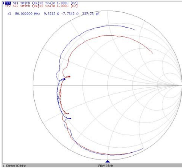
Диаграмма Смита
