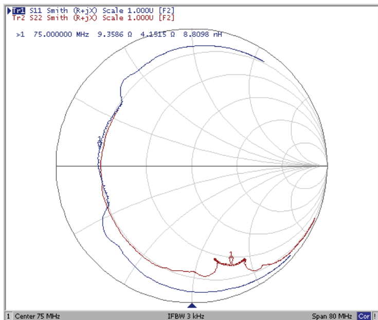
Диаграмма Смита
