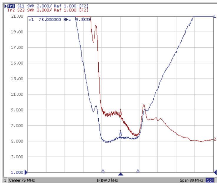
КСВ
