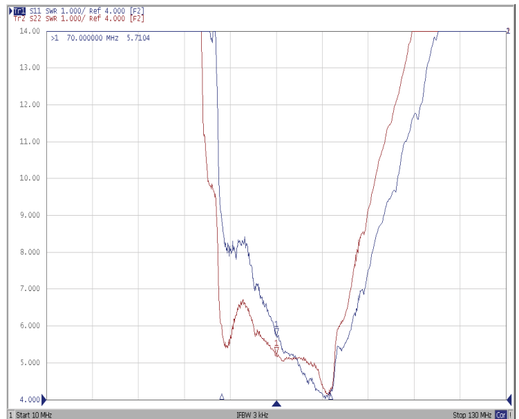
КСВ
