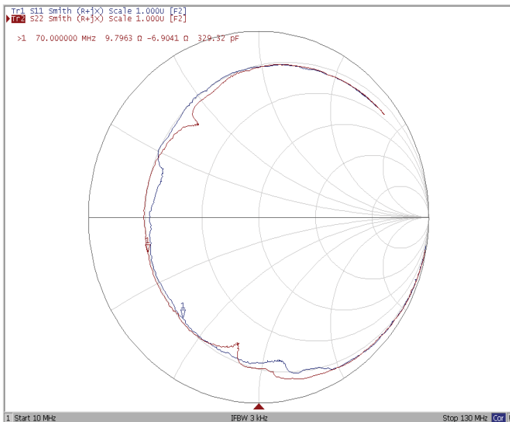
Диаграмма Смита
