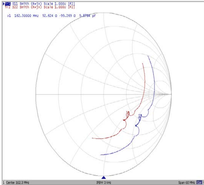
Диаграмма Смита
