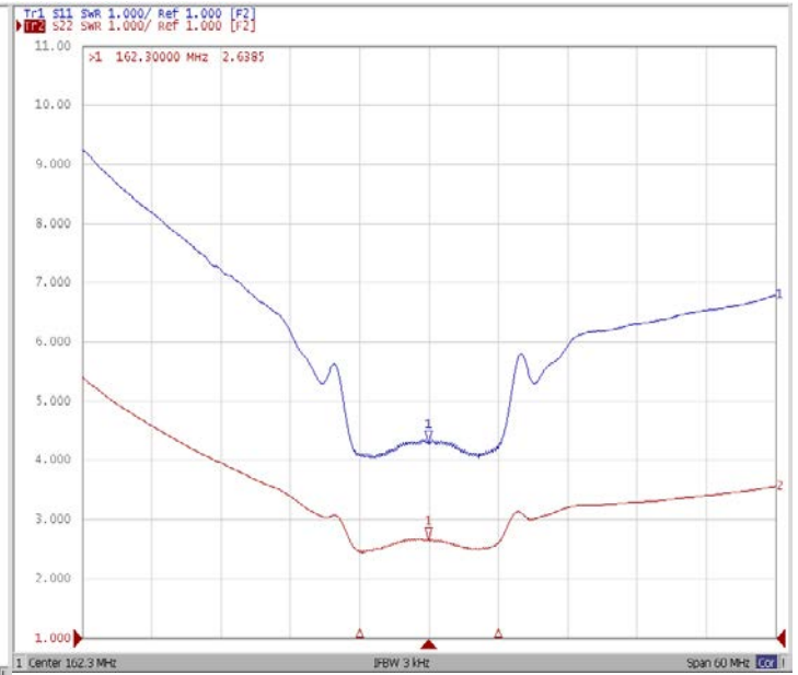
КСВ
