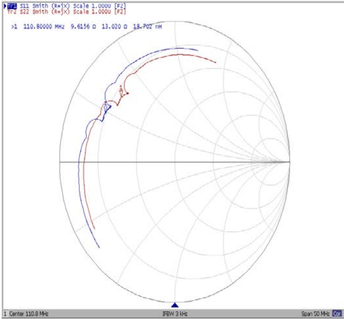
Диаграмма Смита
