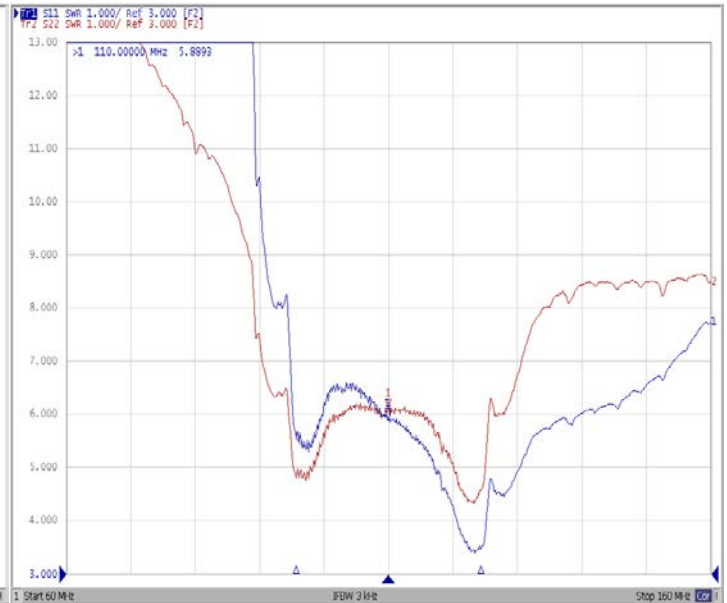
КСВ
