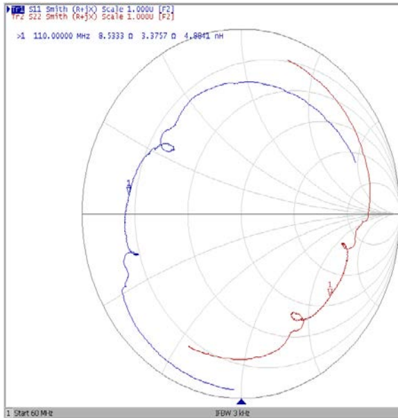
Диаграмма Смита
