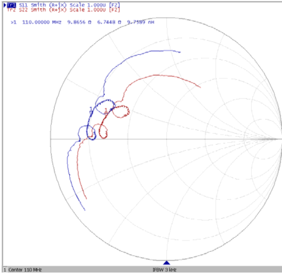
Диаграмма Смита
