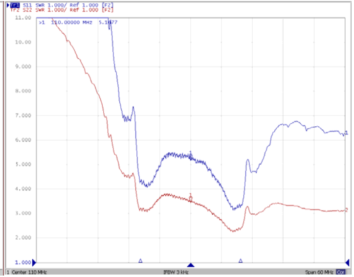
КСВ
