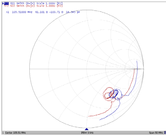
Диаграмма Смита
